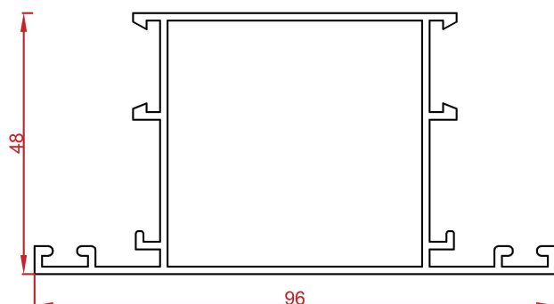
پروفیل سپری T profile Code : 12441 weight : 1.14 kg/m
