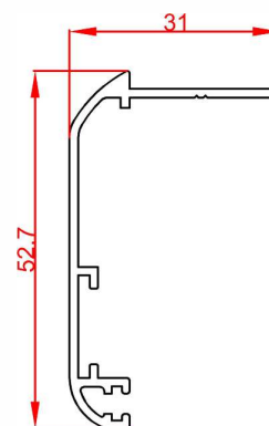
پروفیل روکوب ۵۲
