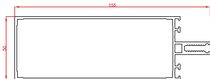
پروفیل افقی Transom profile Code : 53068 weight : 2.19 kg/m
