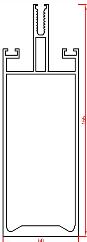
پروفیل عمودی Mullion profile Code : 53064 weight : 3.18 kg/m
