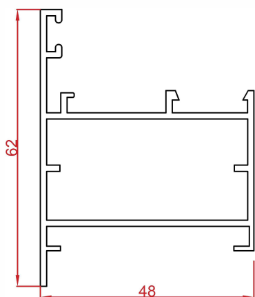
پروفیل فریم Frame profile Code : 14311 weight : 0.99 kg/m
