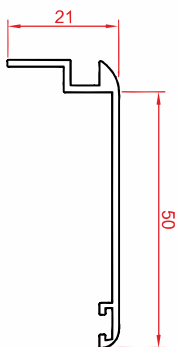
پروفیل روکوب ۴۰ Border profile 40 Code : 10024 weight : 0.25 kg/m
