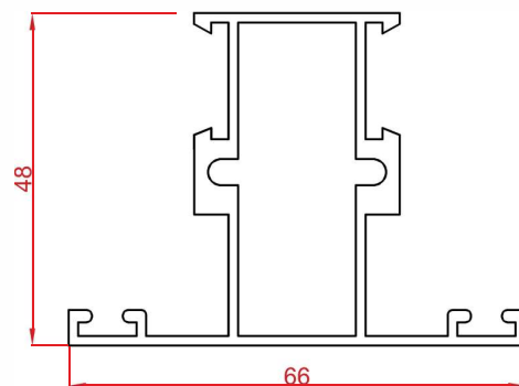
پروفیل سپری T profile Code : 13341 weight : 1 kg/m
