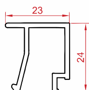
زهوار دو جداره ترمال Double rickety Code : 21351 weight : 0.3 kg/m
