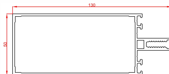
پروفیل افقی Transom profile Code : 53067 weight : 1.87 kg/m
