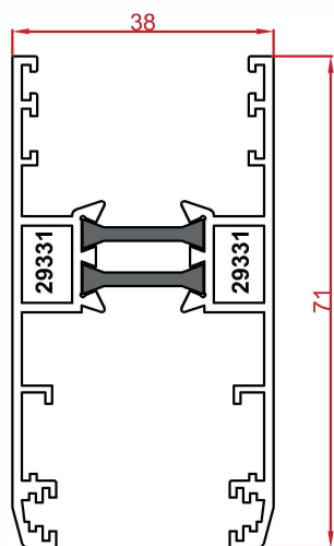
پروفیل لنگه vent profile Code : 29331-29331 weight : 1.15 kg/m
