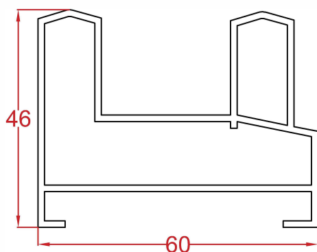
پروفیل فریم Frame profile Code : 15311 weight : 1 kg/m
