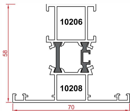
پروفیل سپری T profile Code : 10206-10208 weight : 1.33 kg/m
