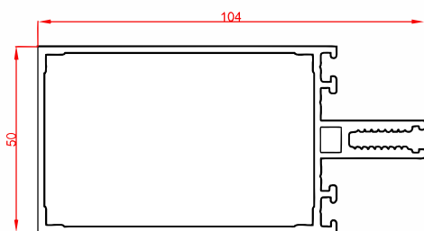
پروفیل افقی Transom profile Code : 53066 weight : 1.67 kg/m
