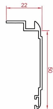
پروفیل روکوب شیاردار ۵۰ Groove Border profile 50 Code : 10027 weight : 0.29 kg/m
