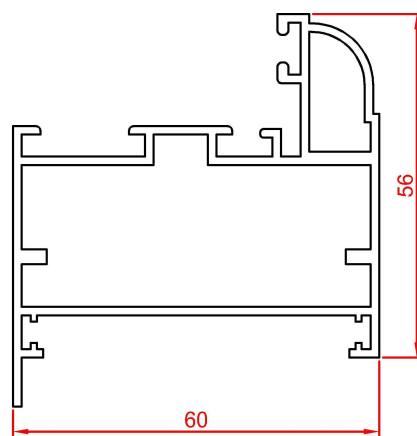
پروفیل فریم Frame profile Code : 13312 weight : 1.17 kg/m
