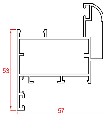
پروفیل لنگه vent profile Code : 13331 weight : 1.11 kg/m
