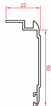
پروفیل روکوب شیاردار ۵۰ Groove Border profile 50 Code : 10027 weight : 0.29 kg/m
