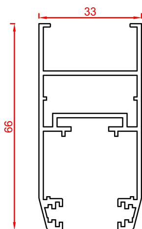
پروفیل لنگه vent profile Code : 15331 weight : 0.92 kg/m
