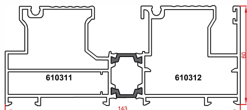
پروفیل فریم Frame profile Code : 610311-610312 weight : 3.41 kg/m
