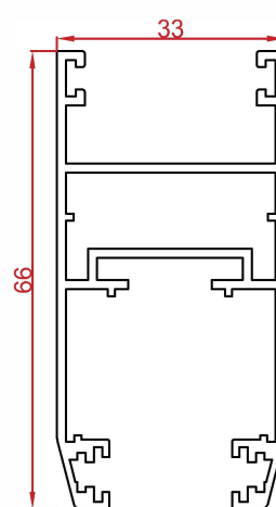
پروفیل لنگه vent profile Code : 15332 weight : 0.93 kg/m
