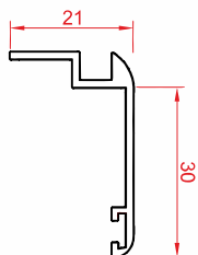
پروفیل روکوب ۳۰ Border profile 30 Code : 10022 weight : 0.22 kg/m
