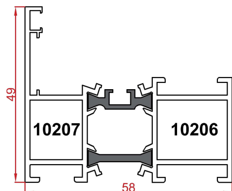
پروفیل فریم Frame profile Code : 10207-10206 weight : 1.2 kg/m
