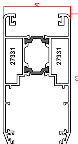
پروفیل لنگه vent profile Code : 27331-27331 weight : 2.12 kg/m
