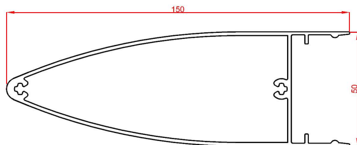
پروفیل درپوش Cap Profile Code : 53024 weight : 1.82 kg/m
