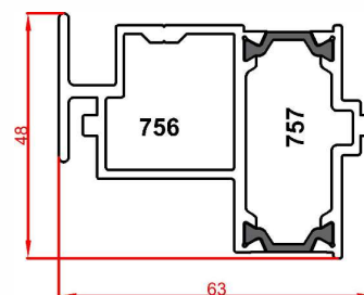
پروفیل وسط چهار لنگه The Middle Four Vent Code : 756-757 weight : 1.6 kg/m
