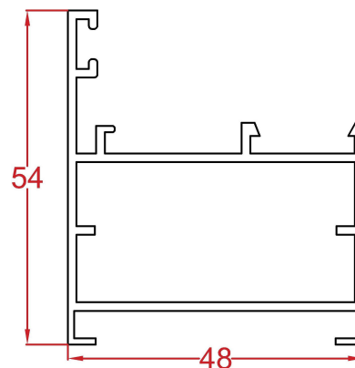
پروفیل فریم Frame profile Code : 12312 weight : 0.8 kg/m
