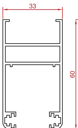
پروفیل لنگه vent profile Code : 15333 weight : 0.8 kg/m
