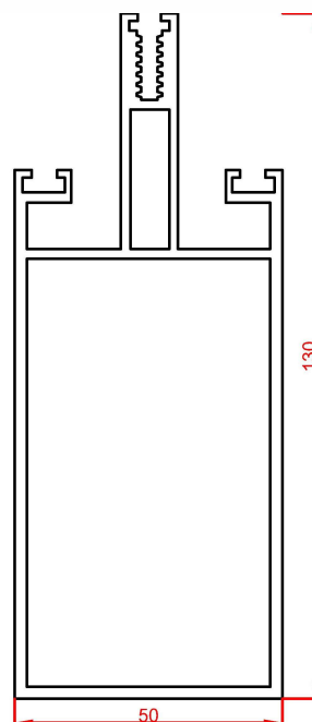
پروفیل عمودی Mullion profile Code : 53061 weight : 2.45 kg/m
