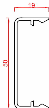
درپوش افقی Transom Cap Code : 53021 weight : 0.35 kg/m
