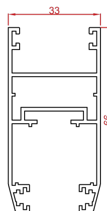
پروفیل لنگه vent profile Code : 15332 weight : 0.93 kg/m
