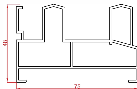
پروفیل فریم Frame profile Code : 16312 weight : 1.29 kg/m
