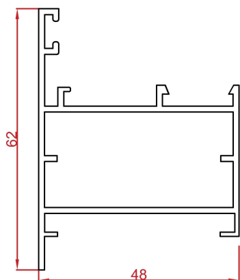
پروفیل فریم Frame profile Code : 12311 weight : 0.84 kg/m
