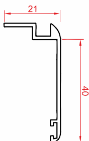
پروفیل روکوب ۴۰ Border profile 40 Code : 10024 weight : 0.25 kg/m
