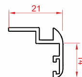
پروفیل روکوب ۱۴ Border profile 14 Code : 10021 weight : 0.2 kg/m
