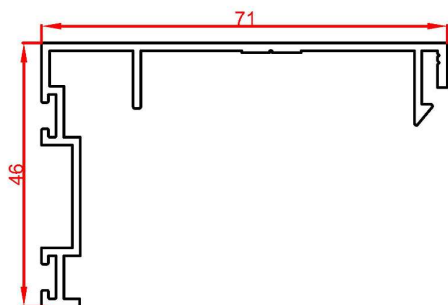
درپوش لنگه
