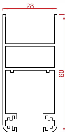
پروفیل لنگه vent profile Code : 14331 weight : 0.8 kg/m
