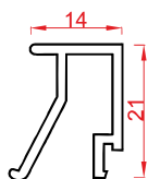
زهوار دو جداره Double rickety Code : 12351 weight : 0.22 kg/m
