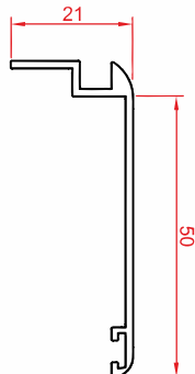
پروفیل روکوب ۵۰ Border profile 50 Code : 10026 weight : 0.28 kg/m
