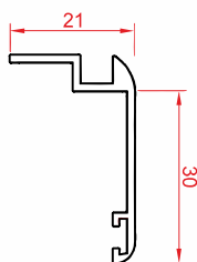
پروفیل روکوب ۳۰ Border profile 30 Code : 10022 weight : 0.22 kg/m
