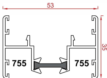
پروفیل وسط چهار لنگه Double rickety Code : 755-755 weight : 0.77 kg/m
