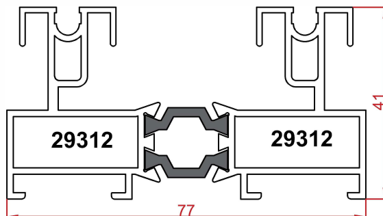
پروفیل فریم Frame profile Code : 29312-29312 weight : 1.6 kg/m
