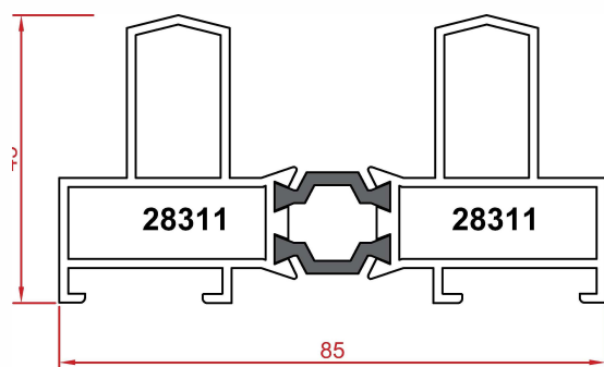
پروفیل فریم Frame profile Code : 28311-28311 weight : 1.65 kg/m
