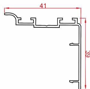
دربوش Gap Code : 28321 weight : 0.27 kg/m
