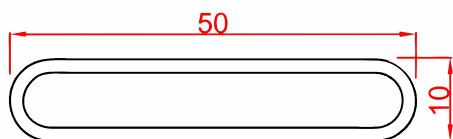
پروفیل گریل Gril Profile Code : 52012 weight : 0.43 kg/m
