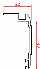
پروفیل روکوب شیاردار ۴۰ Groove Border profile 40 Code : 10025 weight : 0.26 kg/m
