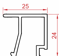
زهوار دو جداره ترمال Double rickety Code : 21352 weight : 0.31 kg/m
