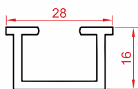
پروفیل شیشه تک جداره Rickety for single glass Code : 14371 weight : 0.35 kg/m
