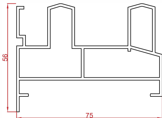
پروفیل فریم Frame profile Code : 16311 weight : 1.32 kg/m
