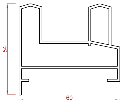
پروفیل فریم Frame profile Code : 15313 weight : 1 kg/m
