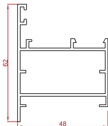
پروفیل فریم Frame profile Code : 12311 weight : 0.84 kg/m
