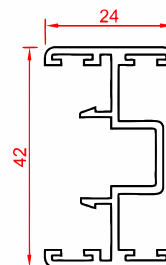
پروفیل وسط چهارلنگه the middle for vent profile Code : 751 weight : 0.5 kg/m
