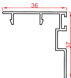
درپوش Gap Code : 15321 weight : 0.26 kg/m
