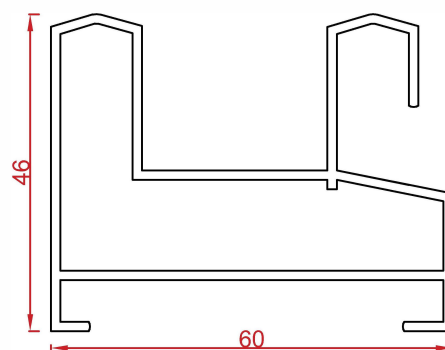
پروفیل فریم Frame profile Code : 15312 weight : 0.98 kg/m
