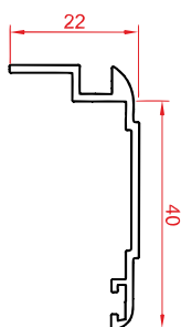
پروفیل روکوب شیاردار ۴۰ Groove Border profile 40 Code : 10025 weight : 0.26 kg/m
