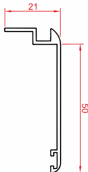
پروفیل روکوب ۵۰ Border profile 50 Code : 10026 weight : 0.28 kg/m
