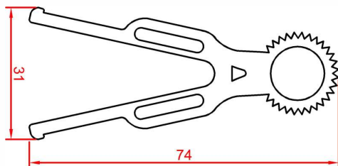
پروفیل پایه متحرک لوور Rotational Louvre Profile Code : 54074 weight : 1.7 kg/m
