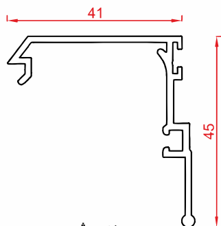
درپوش Gap Code : 29321 weight : 0.43 kg/m
