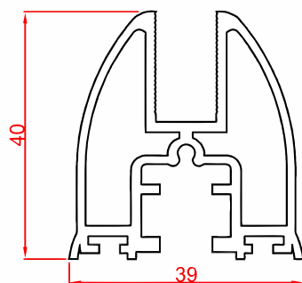
شیشه گیر Glass Stack Code : 56040 weight : 1 kg/m
