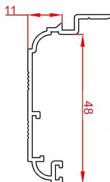
پروفیل روکوب شیاردار ۴۸
