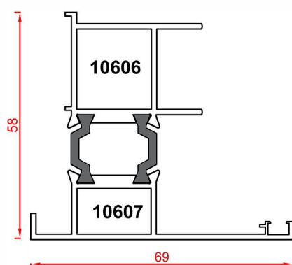
پروفیل وسط دو لنگه the middle of two vent Code : 10606-10607 weight : 1.12 kg/m
