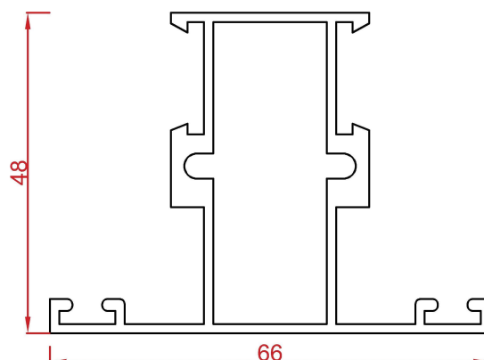
پروفیل سپری T profile Code : 12341 weight : 1 kg/m
