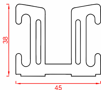
پروفیل لقمه فیکس Fix Piece Profile Code : 53062 weight : 2 kg/m
