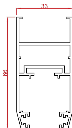
پروفیل لنگه vent profile Code : 15331 weight : 0.92 kg/m
