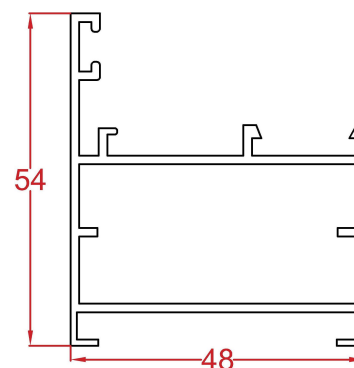
پروفیل فریم Frame profile Code : 12312 weight : 0.8 kg/m
