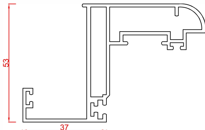
پروفیل دو جداره بازشو Double glazed Opening Profile Code : 51031 weight : 1.25 kg/m
