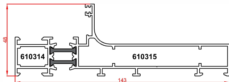
پروفیل کتیبه Engraving profile Code : 610314-610315 weight : 1.48 kg/m
