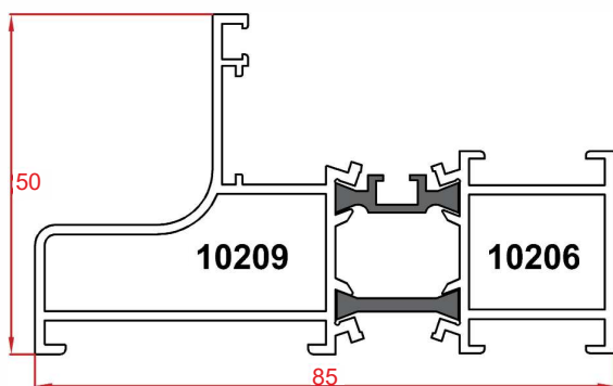
پروفیل فریم Frame profile Code : 10209-10206 weight : 1.42 kg/m
