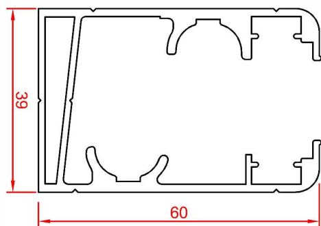
پروفیل ریل Rail Profile Code : 56060 weight : 1.3 kg/m
