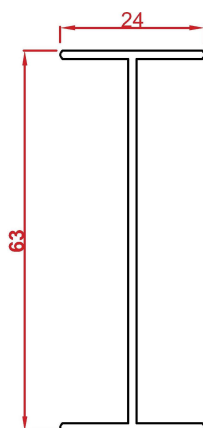
پروفیل وسط ۲ فریم the middle of two frame Code : 752 weight : 0.49 kg/m
