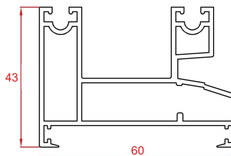
پروفیل فریم Frame profile Code : 15314 weight : 1.12 kg/m
