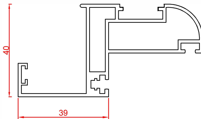
پروفیل دو جداره فیکس Fixed Double Glazing Profile Code : 51011 weight : 1 kg/m
