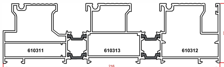
پروفیل فریم سه ریل Frame profile Code : 610311-610313-610312 weight : 5.03 kg/m
