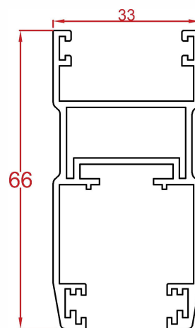
پروفیل لنگه vent profile Code : 15334 weight : 0.94 kg/m
