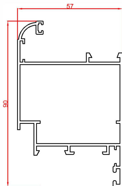
پروفیل لنگه درب vent profile Code : 13332 weight : 1.3 kg/m
