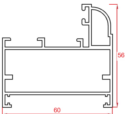
پروفیل فریم Frame profile Code : 13313 weight : 1.14 kg/m
