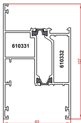
پروفیل لنگه Ventv profile Code : 610331-610332 weight : 2.21 kg/m
