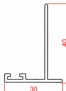
پروفیل پشت نمای بازشو Backside of Opening Faced Profile Code : 51021 weight : 0.3 kg/m
