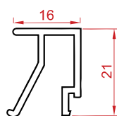
زهوار دو جداره Double rickety Code : 21352 weight : 0.23 kg/m
