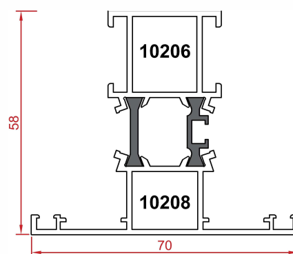
پروفیل سپری T profile Code : 10206-10208 weight : 1.33 kg/m
