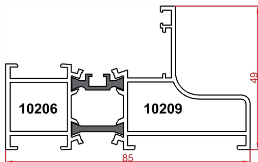
پروفیل فریم Frame profile Code : 10206-10209 weight : 1.42 kg/m
