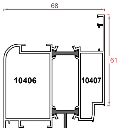
پروفیل لنگه vent profile Code : 10406-10407 weight : 1.8 kg/m
