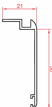
پروفیل روکوب ۵۰ Border profile 50 Code : 10026 weight : 0.28 kg/m
