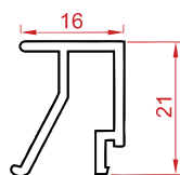
زهوار دو جداره Double rickety Code : 12352 weight : 0.23 kg/m
