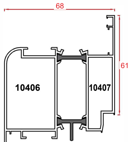
پروفیل لنگه vent profile Code : 10406-10407 weight : 1.8 kg/m
