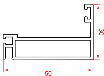
فریم بازشو کرتین وال Curtain Wall Frame Code : 53011 weight : 0.58 kg/m
