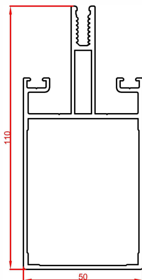
پروفیل عمودی Mullion profile Code : 53063 weight : 1.96 kg/m
