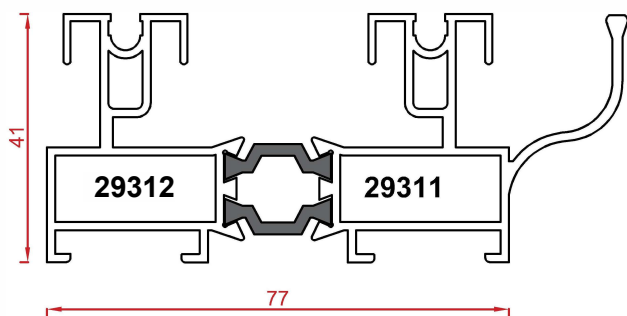
پروفیل فریم Frame profile Code : 29312-29311 weight : 1.75 kg/m
