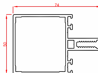
پروفیل افقی Transom profile Code : 53065 weight : 1.38 kg/m
