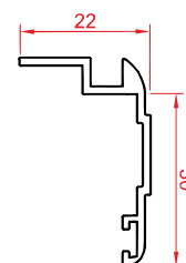
پروفیل روکوب شیاردار ۳۰ Groove Border profile 30 Code : 10023 weight : 0.23 kg/m
