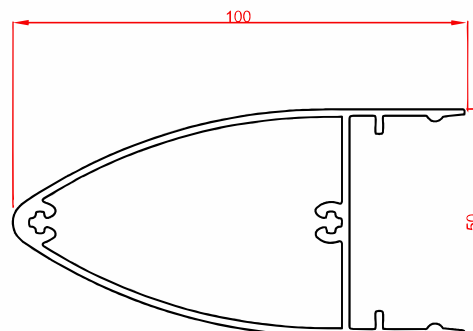
پروفیل درپوش Cap Profile Code : 53023 weight : 1.32 kg/m
