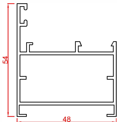
پروفیل فریم بدون لبه Gril Frame Profile Code : 52011 weight : 0.8 kg/m
