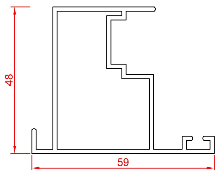
پروفیل وسط دو لنگه Between the two vent profile Code : 12481 weight : 0.84 kg/m
