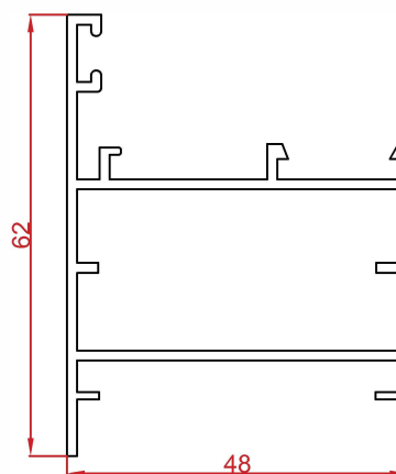
پروفیل کتیبه Engraving profile Code : 12311 weight : 0.84 kg/m
