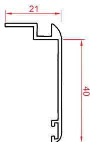
پروفیل روکوب ۴۰ Border profile 40 Code : 10024 weight : 0.25 kg/m
