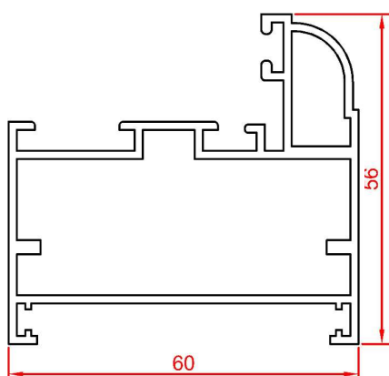
پروفیل فریم Frame profile Code : 13311 weight : 1.14 kg/m
