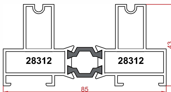
پروفیل فریم Frame profile Code : 28312-28312 weight : 1.57 kg/m
