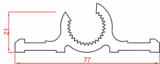
پروفیل پایه ثابت لوور Basic Louvre Profile Code : 54077 weight : 1.55 kg/m
