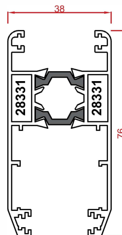
پروفیل لنگه Vent profile Code : 28331-28331 weight : 1.51 kg/m
