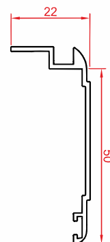
پروفیل روکوب شیاردار ۵۰ Groove Border profile 50 Code : 10027 weight : 0.29 kg/m
