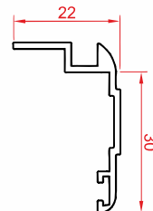
پروفیل روکوب شیاردار ۳۰ Groove Border profile 30 Code : 10023 weight : 0.23 kg/m
