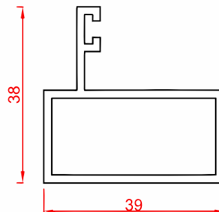
پروفیل کناری Lateral Profile Code : 56038 weight : 0.63 kg/m
