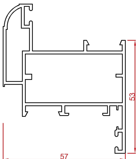
پروفیل لنگه vent profile Code : 12331 weight : 1.1 kg/m
