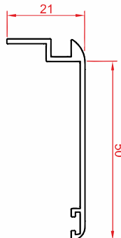
پروفیل روکوب ۵۰ Border profile 50 Code : 10026 weight : 0.28 kg/m
