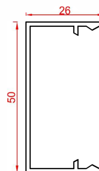
درپوش عمودی Mullion Cap Code : 53022 weight : 0.46 kg/m
