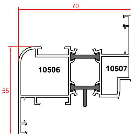
پروفیل لنگه vent profile Code : 10506-10507 weight : 1.49 kg/m
